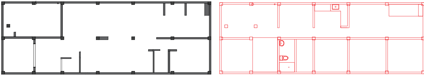
REMODELACION
