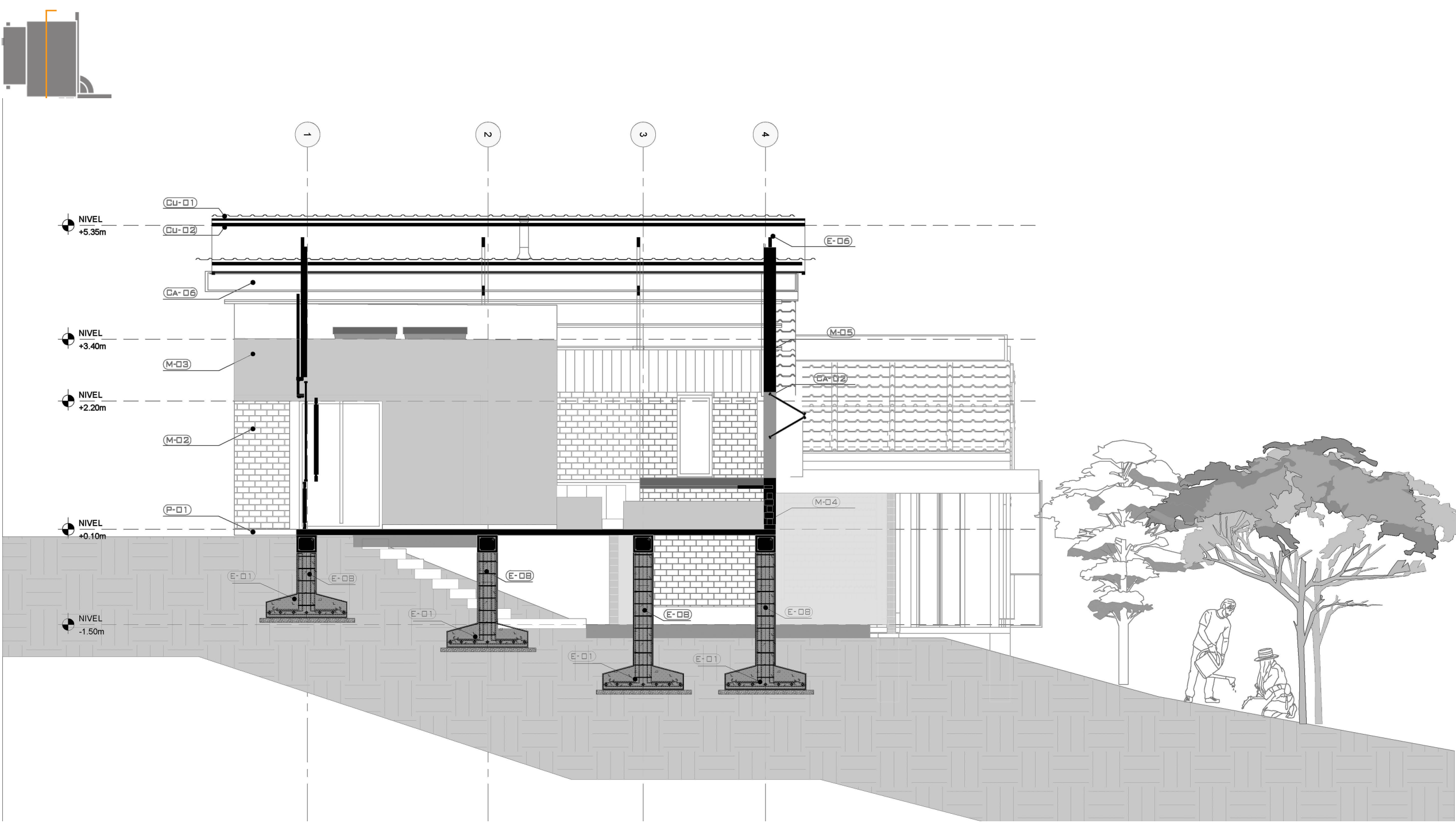
CORTE LONGITUDINAL A-A
