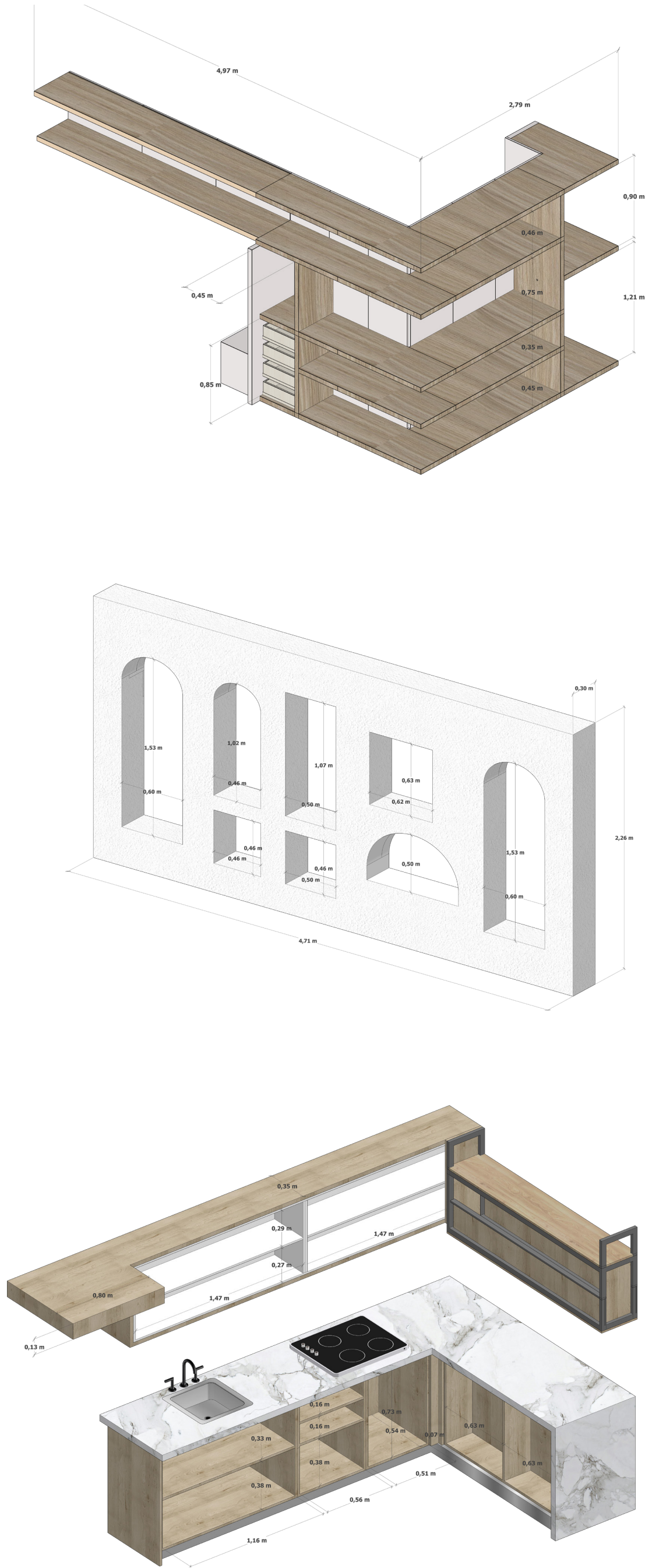
DESPIECE MOBILIARIO
