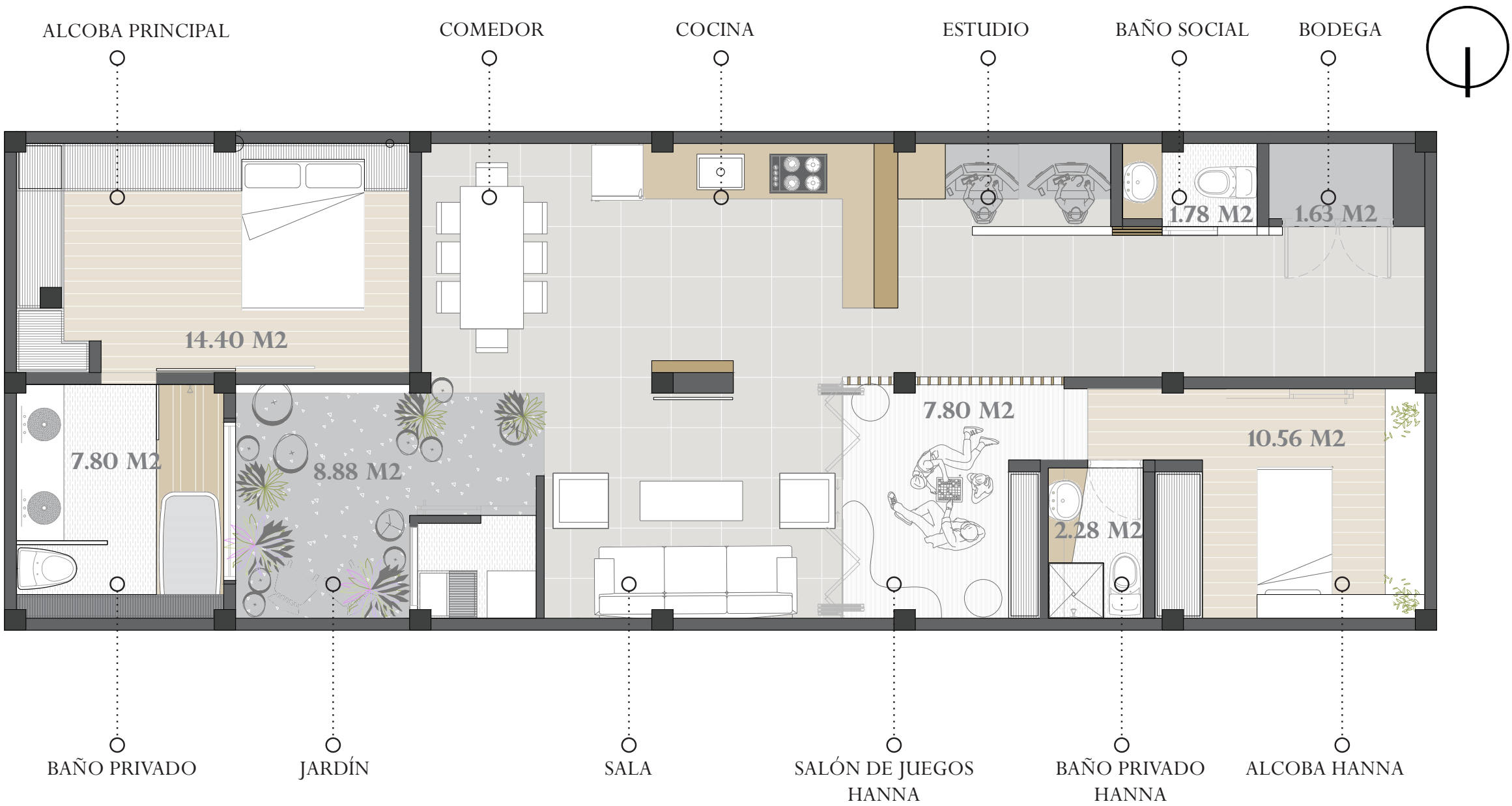
PLANTA ARQUITECTONICA REMODELACION
